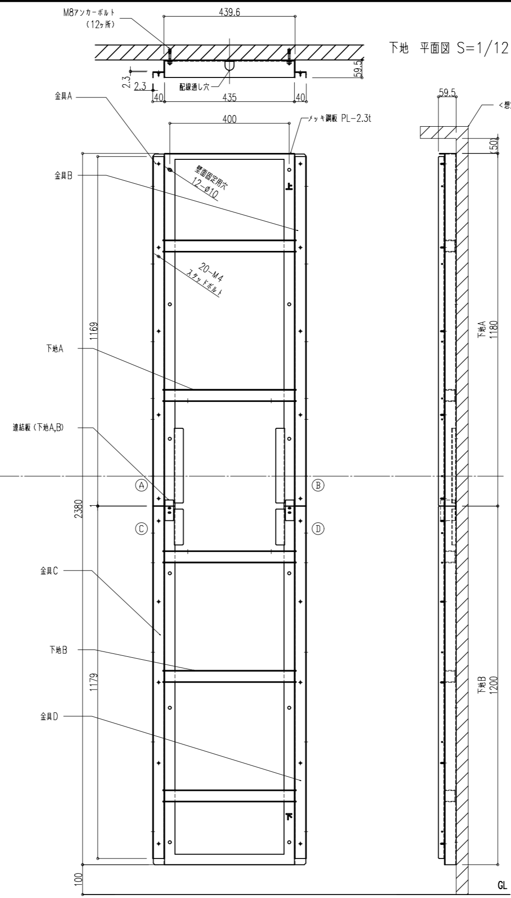
下地 立面図 S=1/12
